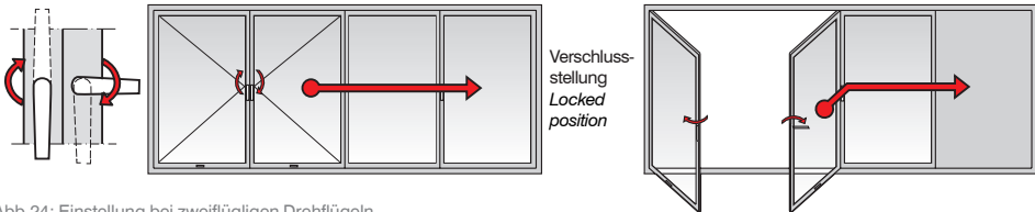
Abb.24: Einstellung bei zweiflügligen Drehflügeln Fig.24: Positions for double leaf casements
